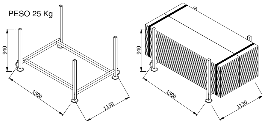
Fig. n. 1
